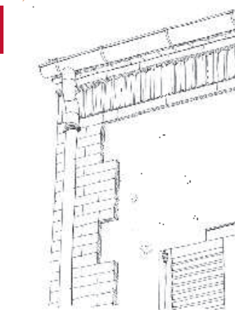
Corniche en dents d'engrenage et chaînage d'angle en brique structurant la façade en moellon
