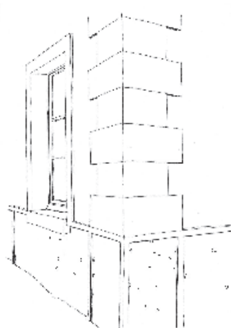
Le tableau de la fenêtre est traité de la même façon que le chaînage d'angle, simplement exécutés en enduit, lissé et de plus forte épaisseur que celui protégeant la façade. Le soubassement en rocaillage reste apparent
