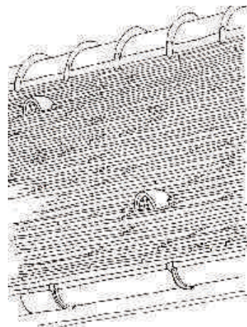
Ventilation sur une toiture en tuile plate par des éléments discrets (chatières) réparties en quinconce, alternativement en haut et en bas des rampants
