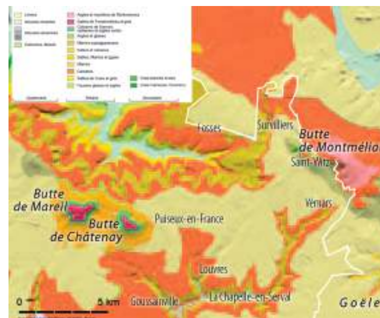
CARTE GÉOLOGIQUE
