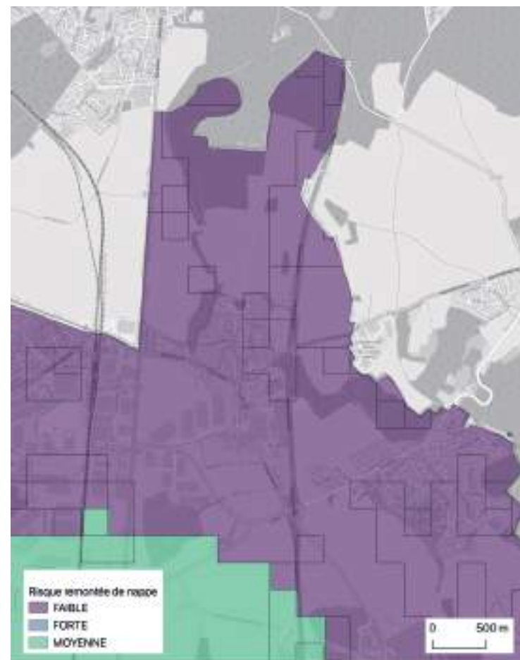
RISQUE DE REMONTÉE DE NAPPE
