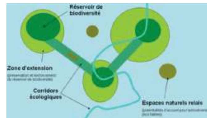
SCHÉMATISATION DE LA NOTION DE CONTINUITÉ ÉCOLOGIQUE
