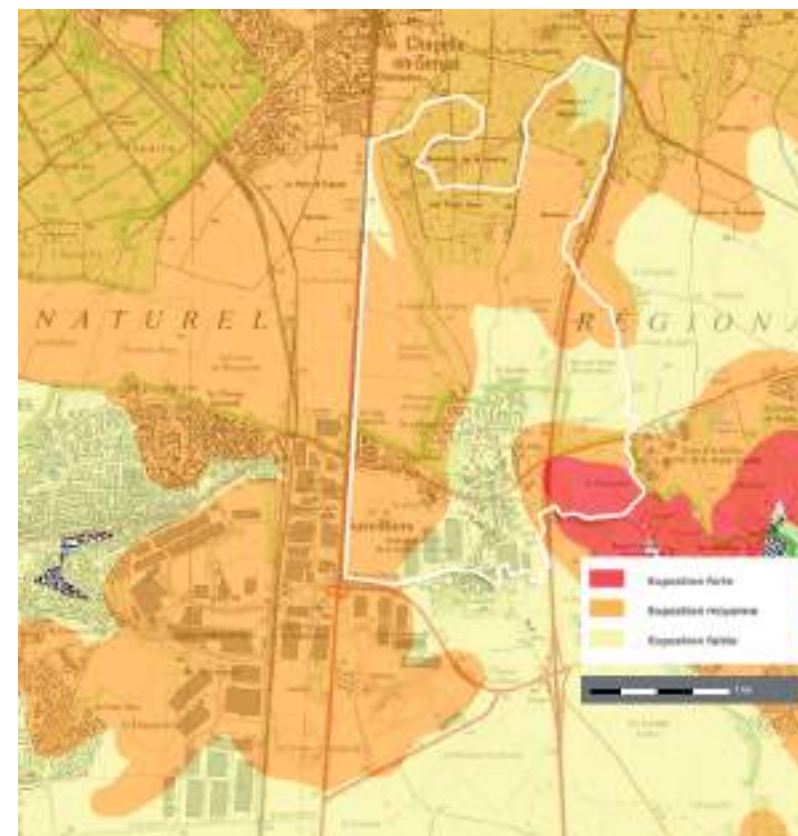
RISQUE DE RETRAIT-GONFLEMENT DES ARGILES
